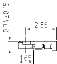
MURATA JSC DETAIL
